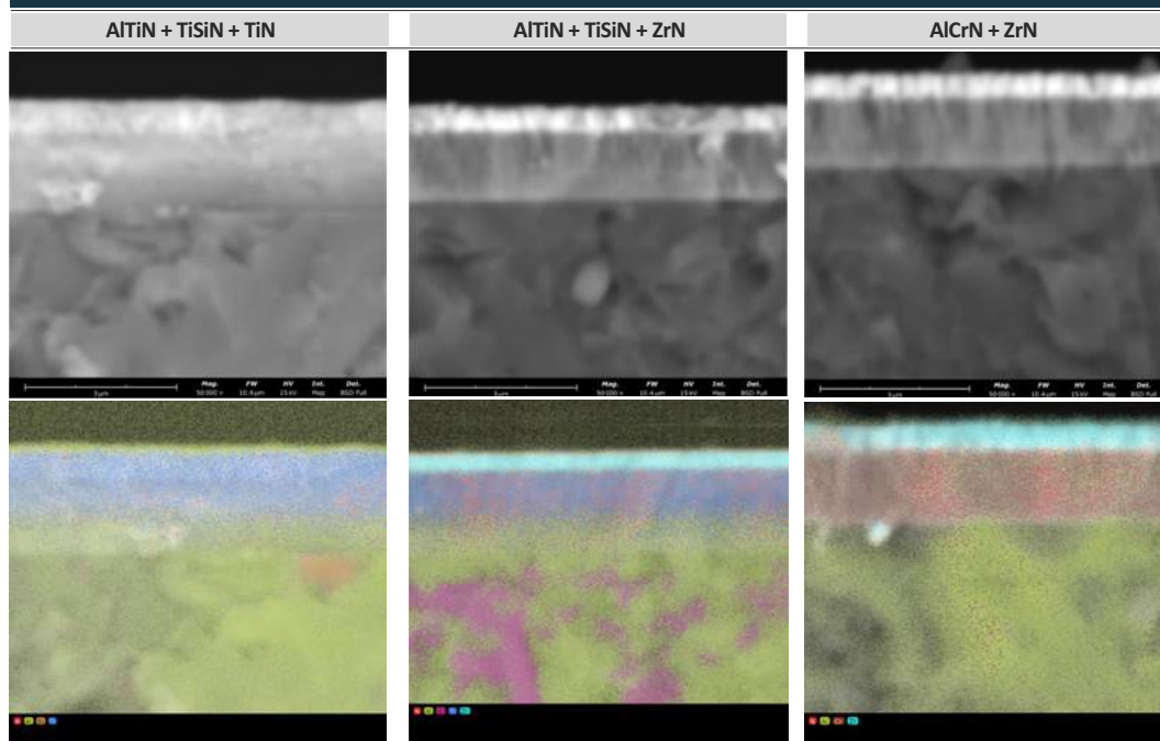
FIGURA 5 Imagens SEM e mapas de distribuição elemental EDS das secções transversais dos três sistemas de revestimento.
