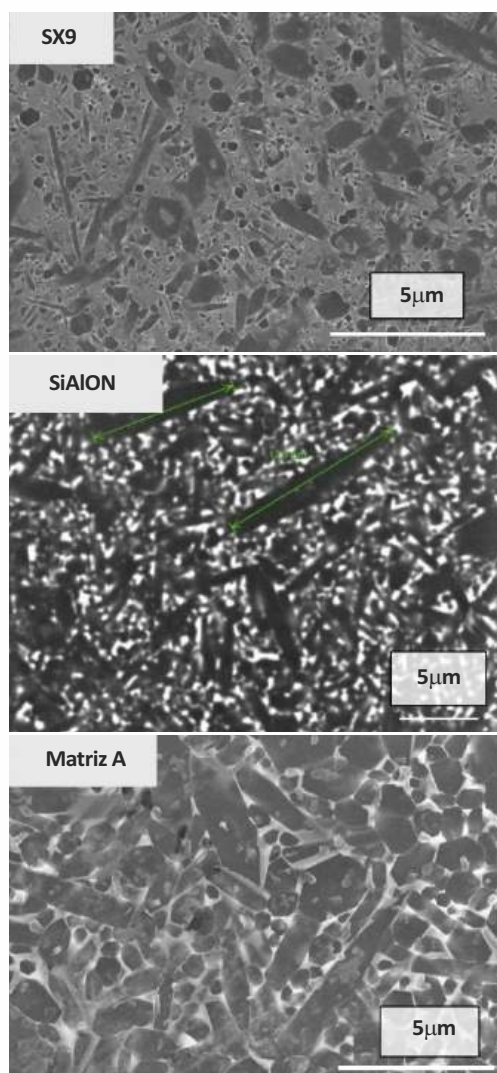
FIGURA 2 Micrografias das amostras SX9, SiAlON e Matriz A.
