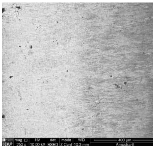
FIGURA 5 Imagens SEM da superfície do inserto após revestimento T6.
