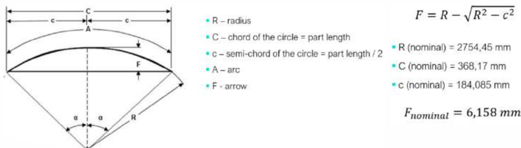
FIGURA 5 Método de correlacionamento das medições (ISRA vs. Blue Laser).
