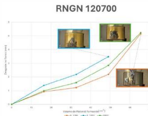
FIGURA 3 Desgaste no flanco VS Volume de Material Removido para geometria RNGN 120700.
