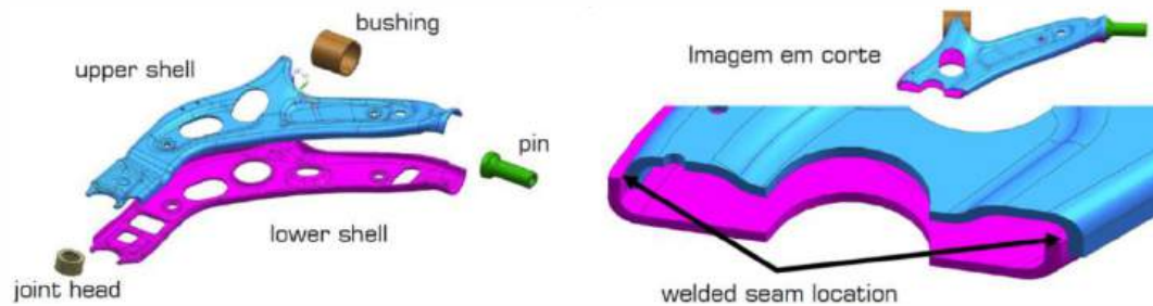
FIGURA 2 Vista explodida do braço de suspensão.
