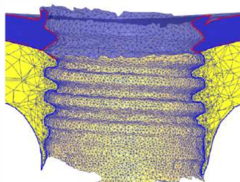
FIGURA 12 Influência do tamanho inicial dos elementos de malha no processo de remeshing: rosca formada - malha inicial 0.1 mm.
