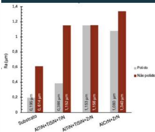
FIGURA 3 Rugosidade superficial das amostras no estado polido e retificado, obtido por microscopia digital.
