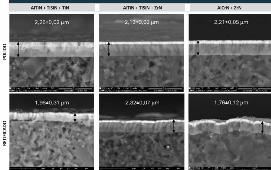
FIGURA 4 Imagens SEM da secção transversal dos diferentes sistemas de revestimento no estado polido e retificado.
