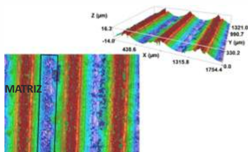
FIGURA 3 Levantamento de forma da ranhura.
