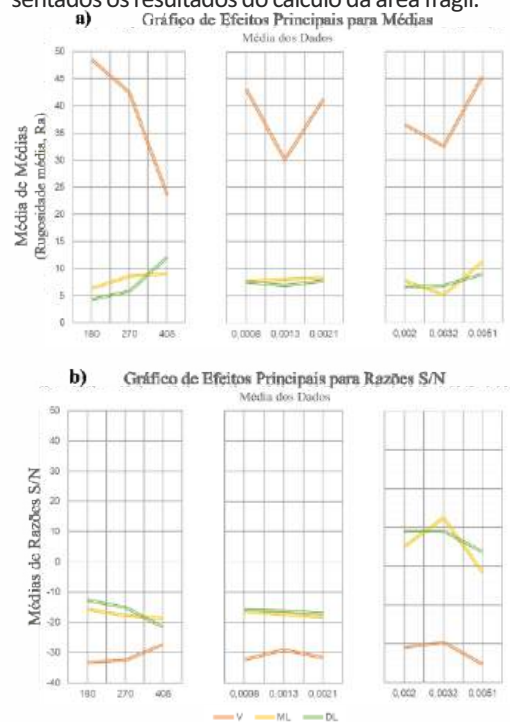
FIGURA 5 Cálculo % área frágil, análise Taguchi com a) gráfico de efeitos principais para médias, b) gráfico de efeitos principais para razões S/N.
