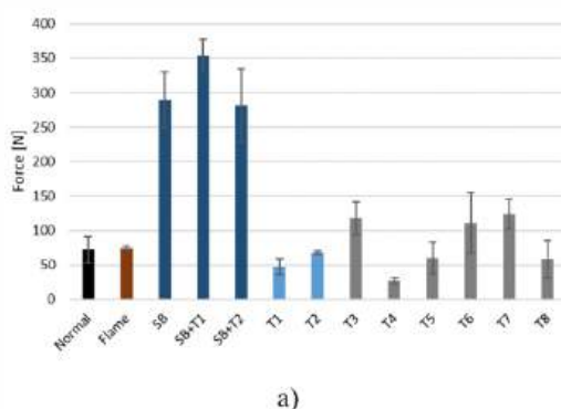
FIGURA 3 a) força máxima registada durante o ensaio de tração; b) rugosidade média dos pinos após tratamento.
