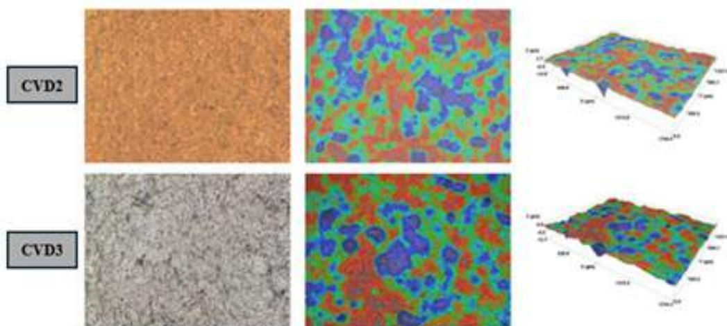
FIGURA 4 Imagens de perfilometria ótica das amostras CVD2 e CVD3
