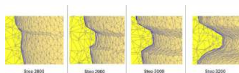
FIGURA 14 Formação da rosca ao longo dos intervalos de tempo - software DEFORM.
