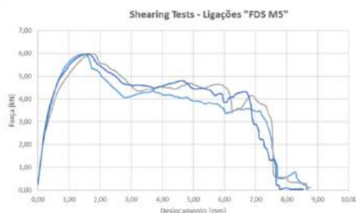
FIGURA 10 Resultados dos ensaios de tração (shearing tests): gráfico Força-Deslocamento.
