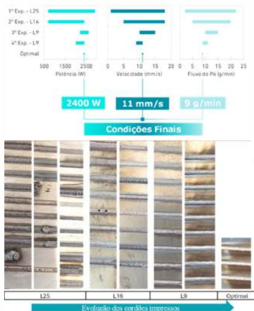
FIGURA 4 Plano experimental para escolher o melhor parâmetro DED.
