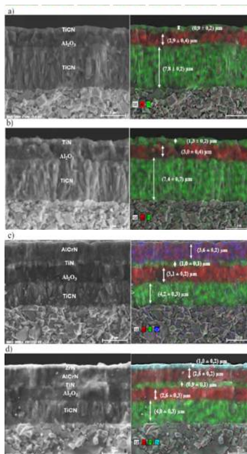
FIGURA 2 Imagens SEM e SEM-EDS do revestimento multicamada (corte transverso) das amostras CVD1 (a), CVD2 (b), CVD3 (c) e CVD4 (d).
