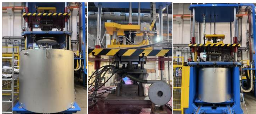
FIGURA 1 Equipamento de fundição por baixa pressão - fases do processo.
