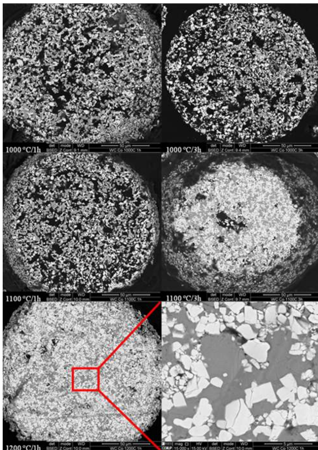
FIGURA 3 Observação feita por SEM nas secções transversais dos grânulos que ilustram a densificação do pó a diferentes temperaturas/tempos.
