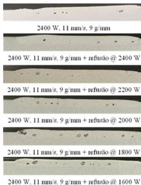
FIGURA 6 Evolução das porosidades em função da potência do laser na refusão.
