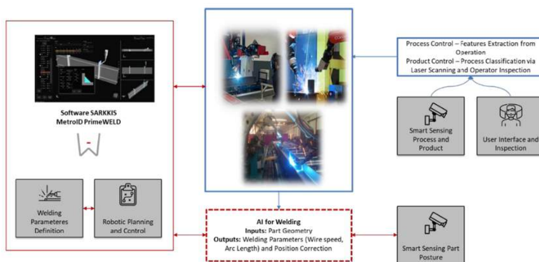
FIGURA 1 Diagrama de funcionamento.
