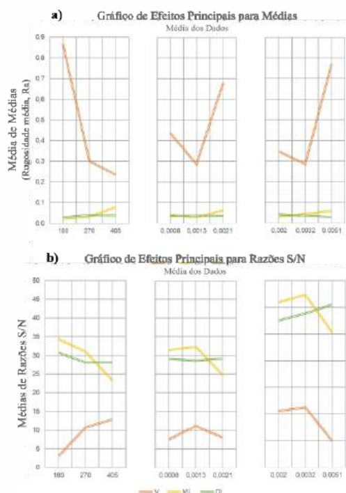
FIGURA 4 Rugosidade média R_a , análise Taguchi com a) gráfico de efeitos principais para médias, b) gráfico de efeitos principais para razões S/N.
