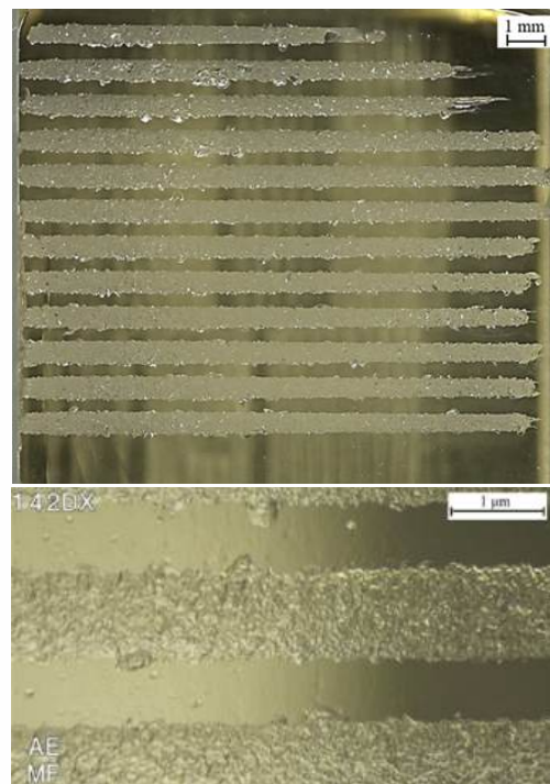
FIGURA 6 Ranhuras maquinadas na condição de inclinação nula ( 0^\circ ), no vidro.
