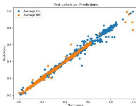
FIGURA 5 Gráfico com a previsão do modelo Random Forest vs previsão esperada.
