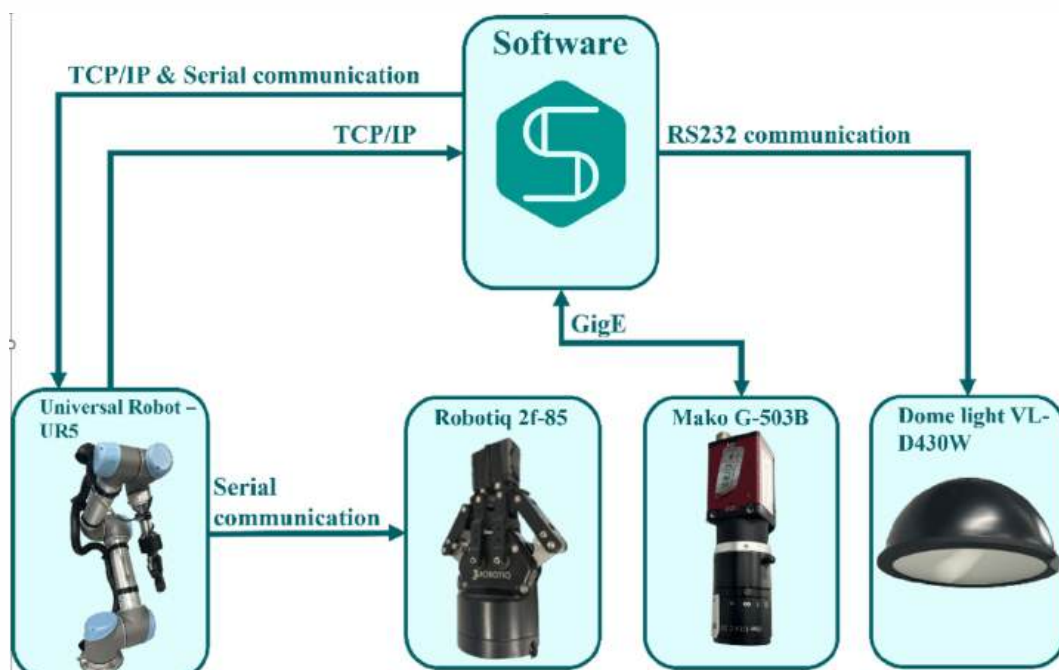
FIGURA 4 Diagrama de blocos da arquitectura do sistema de inspeção.
