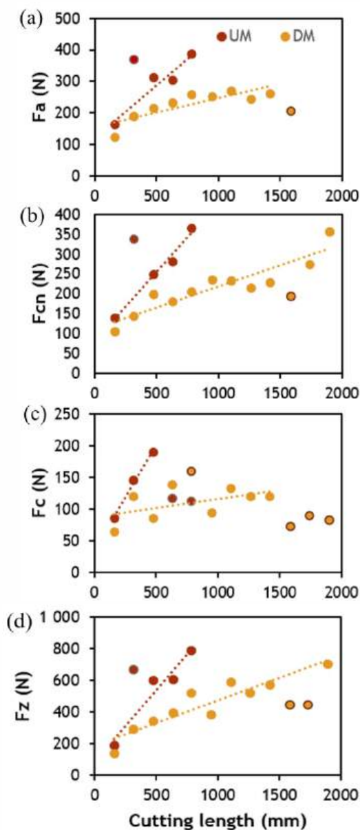
FIGURA 3 Forças de corte registadas para o modo de fresagem discordante (UM) e concordante (DM) para as diferentes componentes: F_a (a); F_c (b); F_{cn} (c) e F_z (d).
