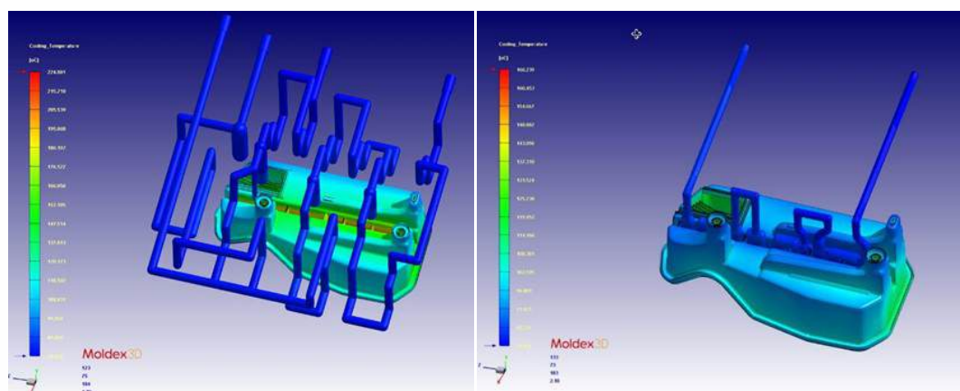
FIGURA 2 Simulação de variação térmica entre circuitos de águas do caso de estudo: Circuito de águas convencional (a), Circuito com canais conformais (b).
