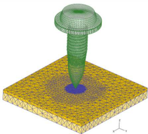
FIGURA 3 Modelo do FDS construído pelo método dos elementos finitos recorrendo as software DEFORM 3D.
