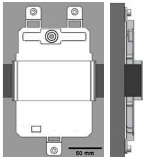
FIGURA 4 Vista superior e lateral da peça depois da operação de facejamento.
