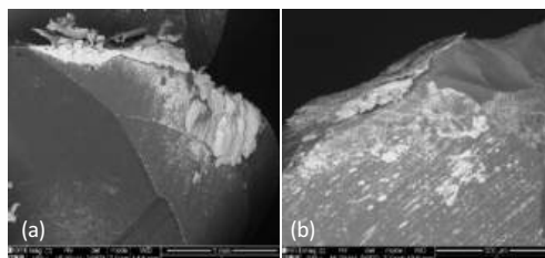
FIGURA 5 Mecanismos de desgaste observados nas ferramentas testadas: adesão de material no flanco gume de corte (a); destacamento do substrato (cratera) e adesão de material à superfície da ferramenta (b).
