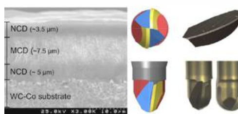
FIGURA 1 Revestimento e geometria da ferramenta.
