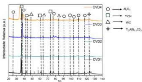
FIGURA 3 Difractogramas de raios X das amostras
