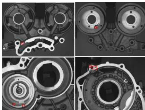
FIGURA 2 Exemplos de porosidade na superfície das peças.
