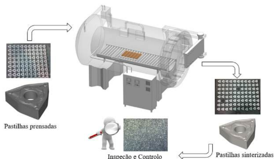
FIGURA 2 Exemplificação das peças prensadas e sinterizadas.
