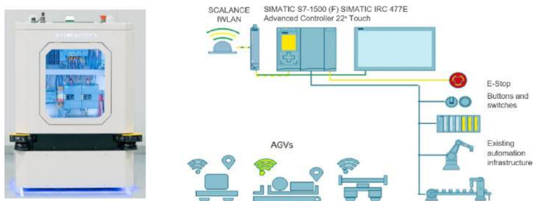
FIGURA 1 Estrutura de comunicação Factory - Machine
