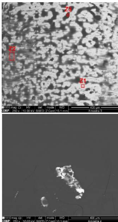
FIGURA 4 Imagens SEM da superfície dos pinos após tratamento: a) T3; b) T4
