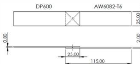
FIGURA 3 Geometria e dimensões da junta aparafusada.
