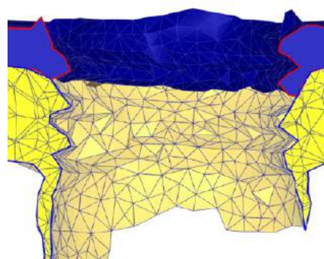
FIGURA 13 Influência do tamanho inicial dos elementos de malha no processo de remeshing: rosca formada - malha inicial 0.5 mm.
