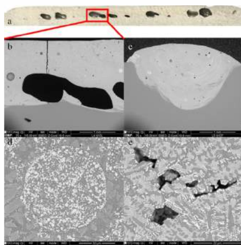
FIGURA 5 Observação de defeitos das secções longitudinais e transversais da linha impressa com 2400 W, 11 mm/s e 9 g/min.
