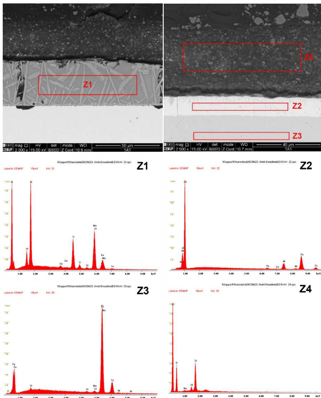
FIGURA 6 Análise dos elementos químicos presentes na amostra 1A-I.
