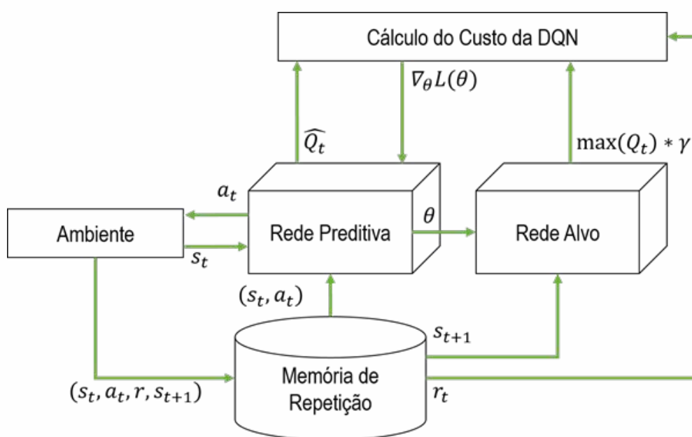
FIGURA 1 Diagrama de blocos para DQN.
