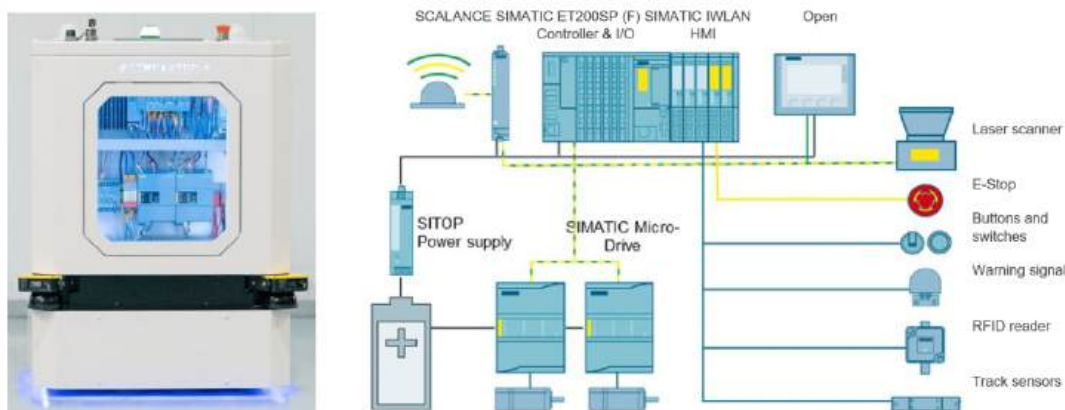
FIGURA 2 Arquitetura lógica do Streaktec-1.
