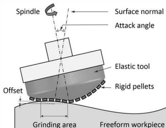
FIGURA 1 Princípio das ferramentas de retificação adaptativa à forma [1].
