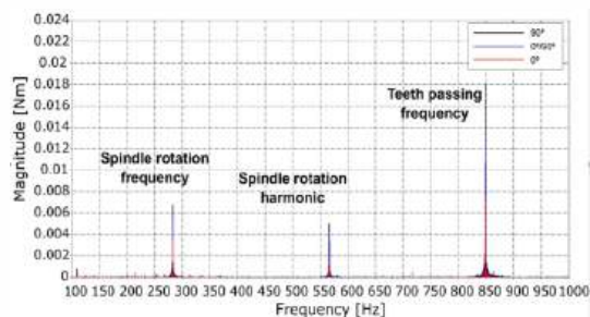
FIGURA 2 FFT do sinal do momento M_z .
