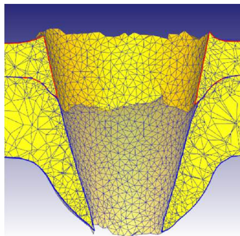
FIGURA 4 Modelação das chapas após penetração.
