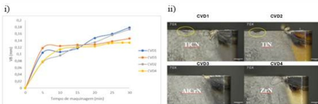
FIGURA 5 i) Desgaste do flanco em função do tempo de maquinagem v_b ; ii) Imagens capturadas com microscópio ótico das amostras após maquinagem de 30 minutos.
