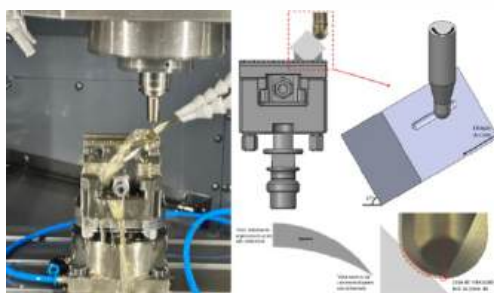
FIGURA 2 Representação da montagem experimental.
