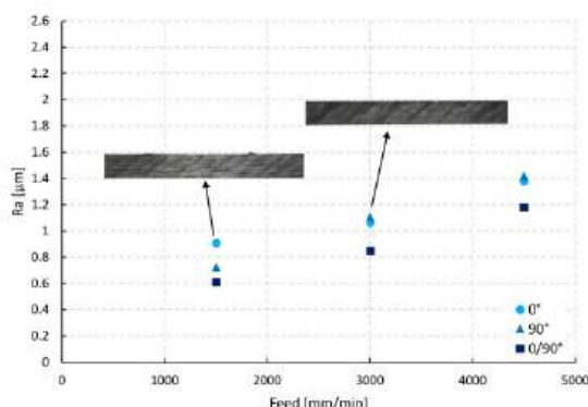
FIGURA 5 Rugosidade média em função do avanço e ângulo de corte das fibras.
