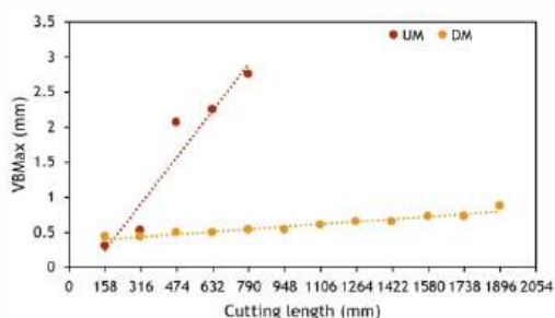
FIGURA 4 Desgaste de flanco (VB) medido nas ferramentas após maquinagem, ao longo da distância maquinada.
